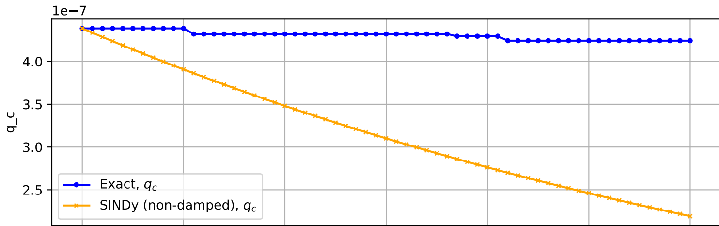
Trajectory No. 3434
