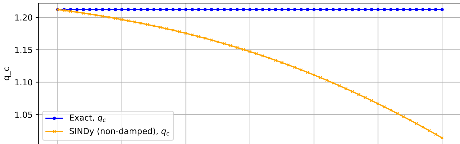
Trajectory No. 3448
