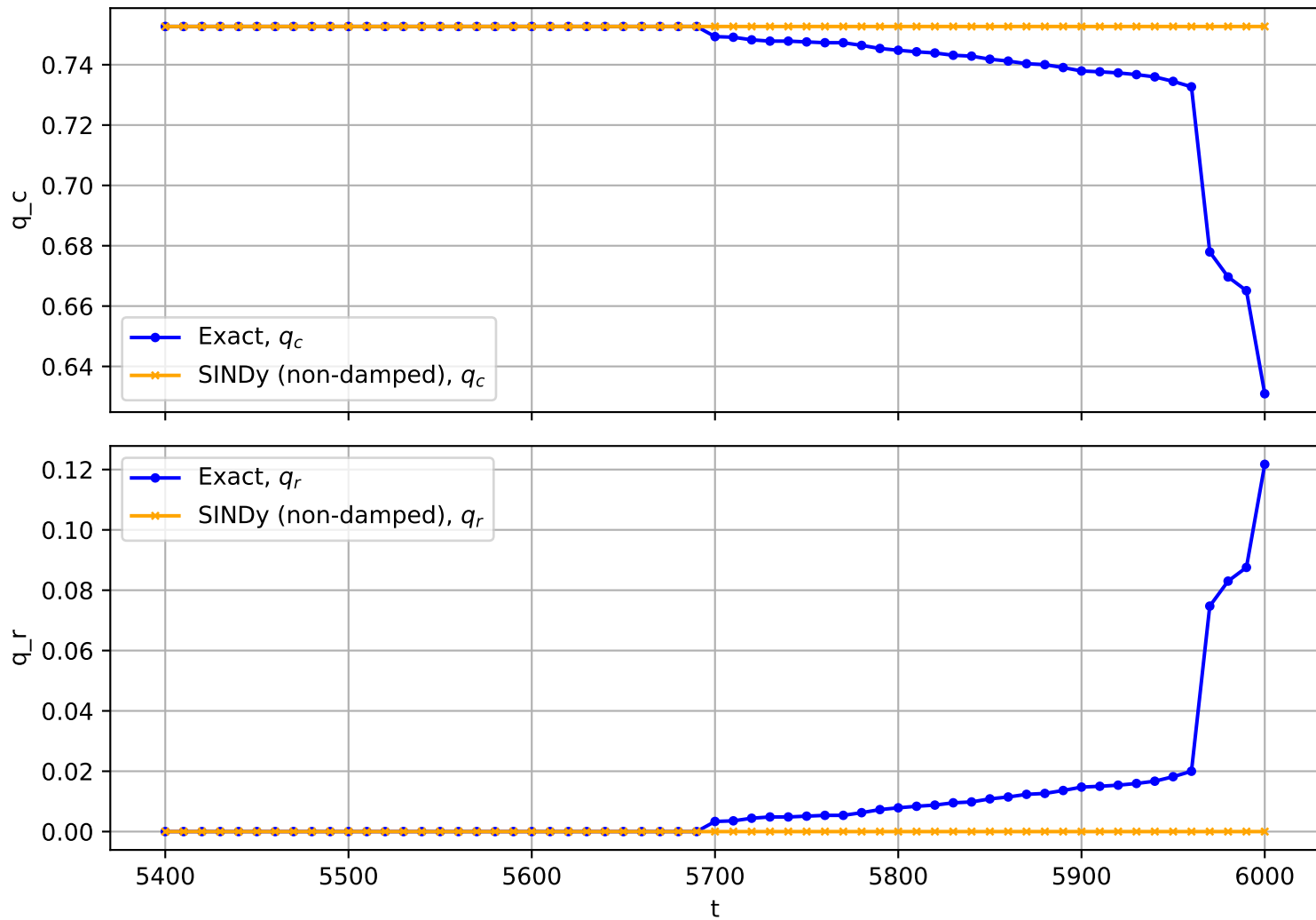
Trajectory No. 3487
