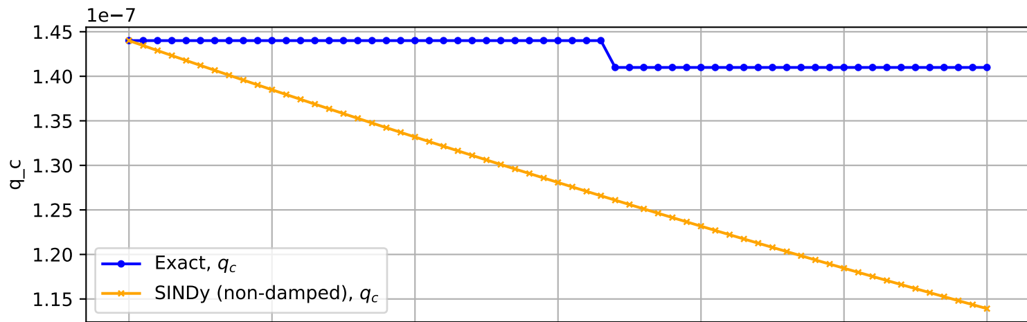
Trajectory No. 3491
