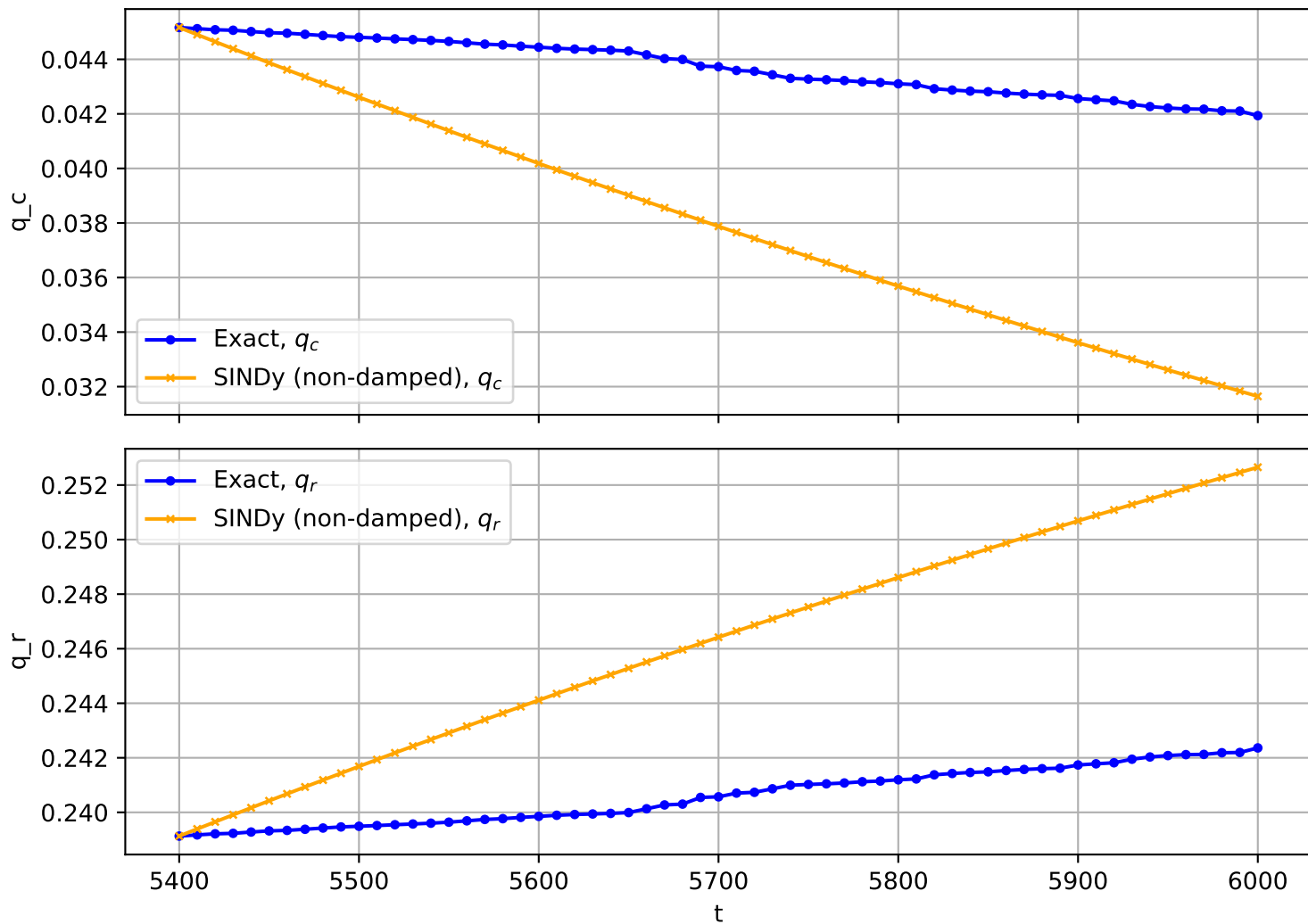
Trajectory No. 461
