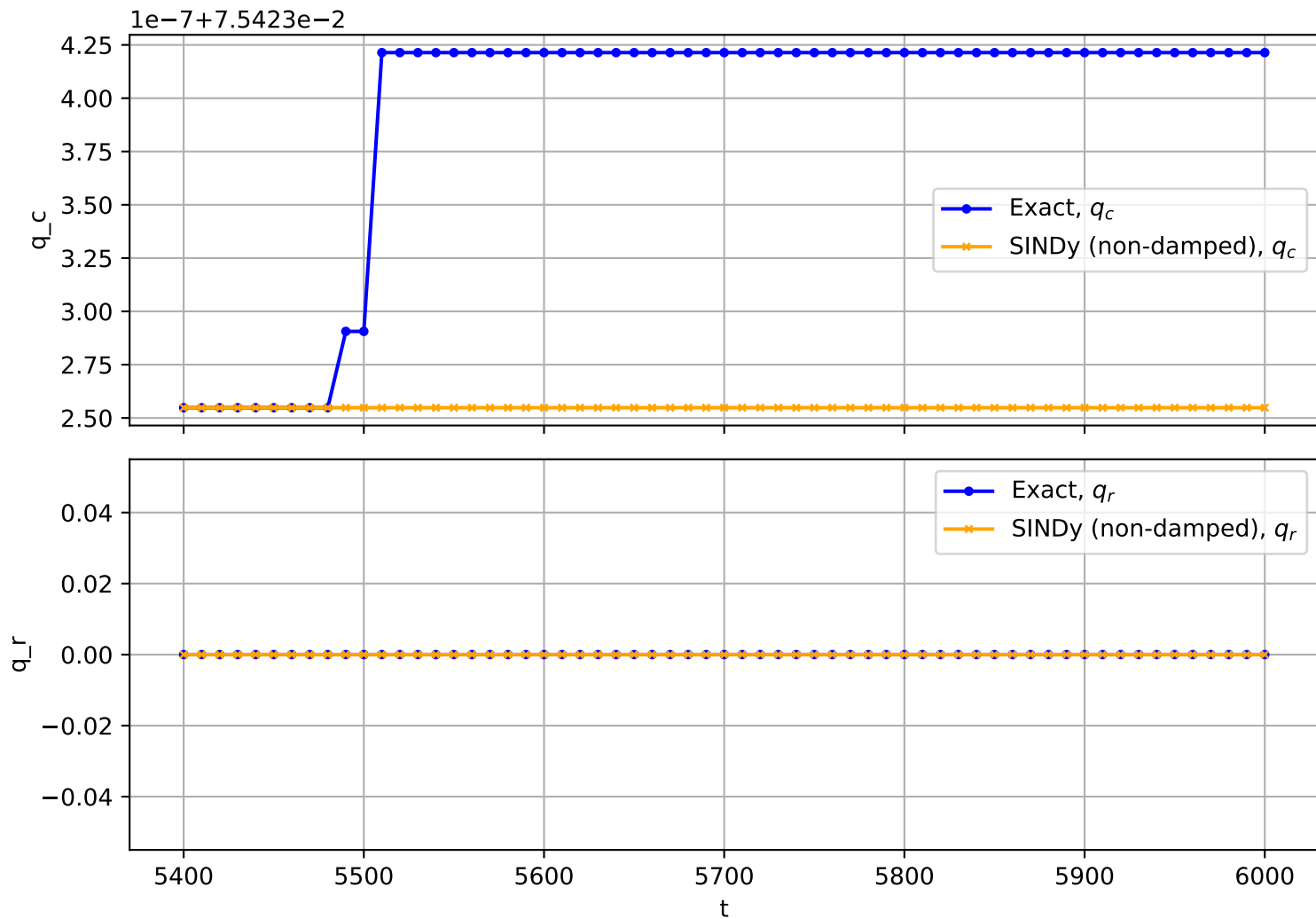
Trajectory No. 518
