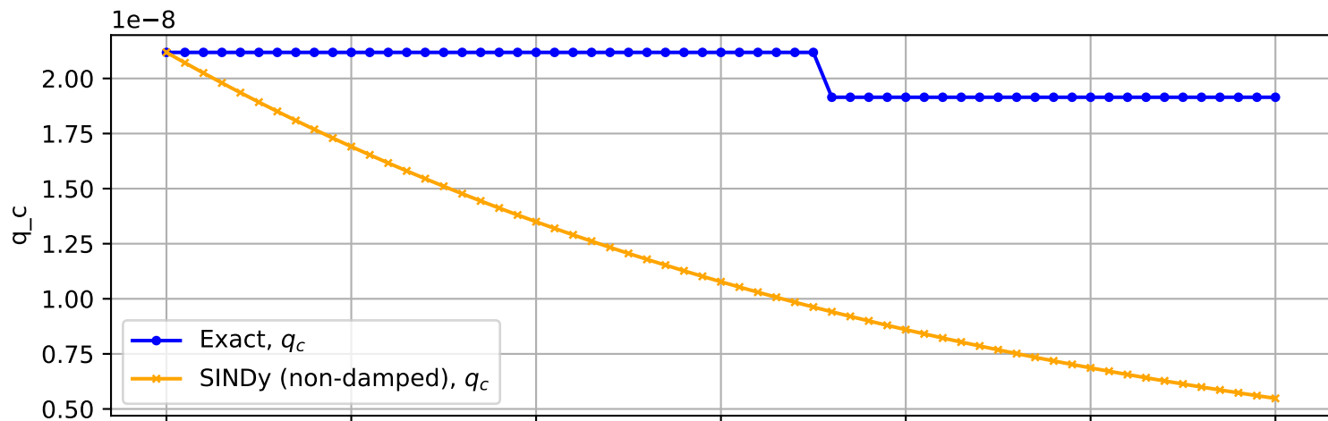
Trajectory No. 575
