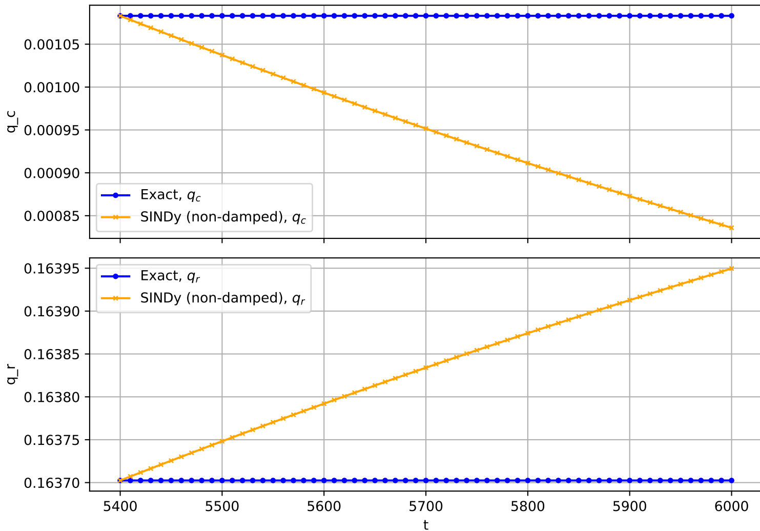
Trajectory No. 602
