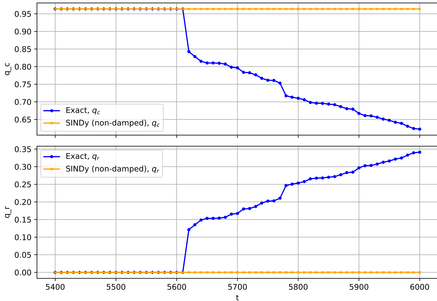
Trajectory No. 616
