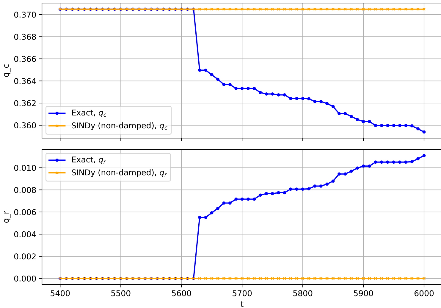
Trajectory No. 619
