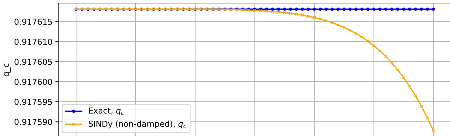
Trajectory No. 625
