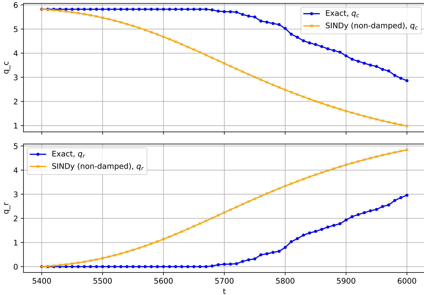
Trajectory No. 645
