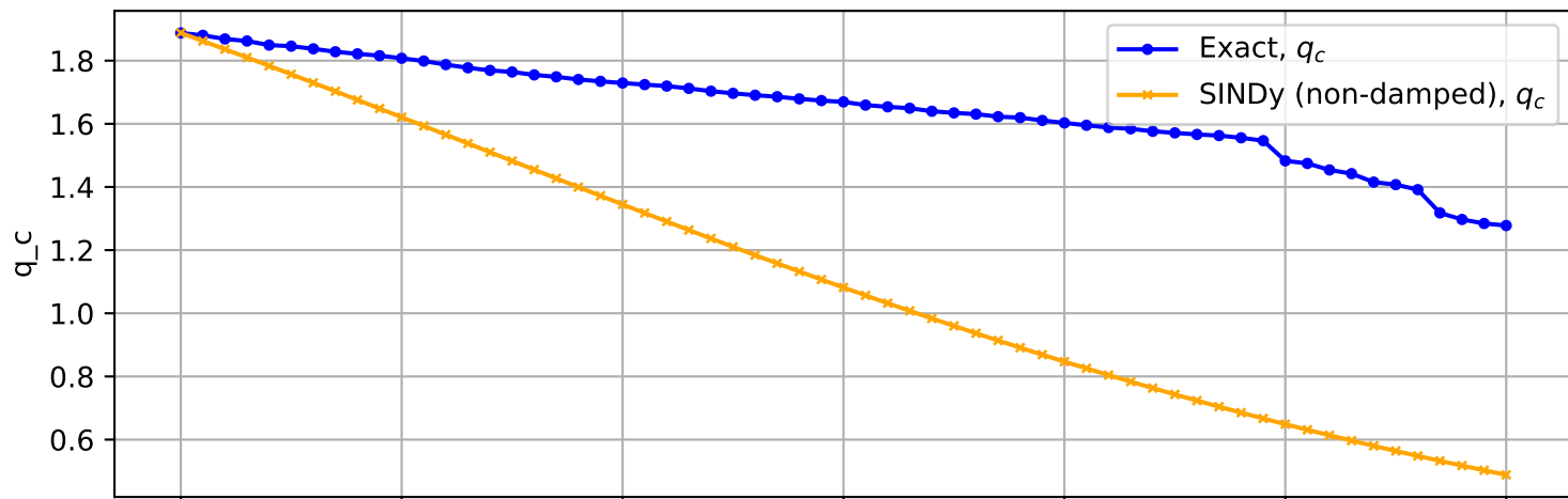
Trajectory No. 711
