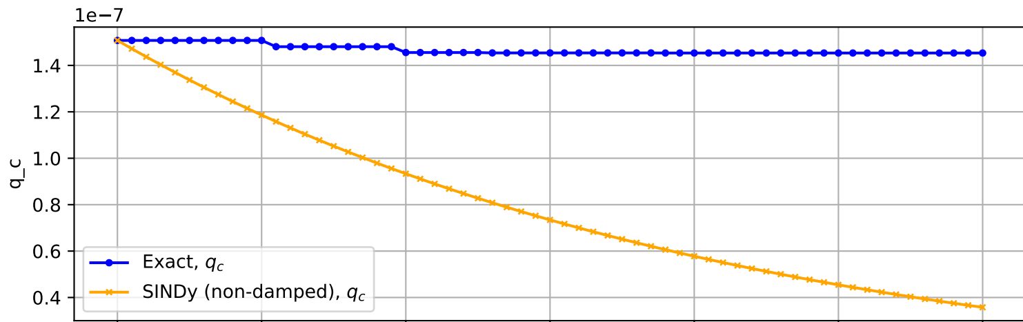
Trajectory No. 721
