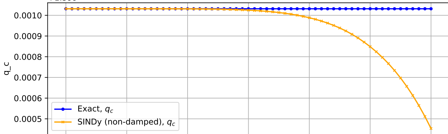
Trajectory No. 786
