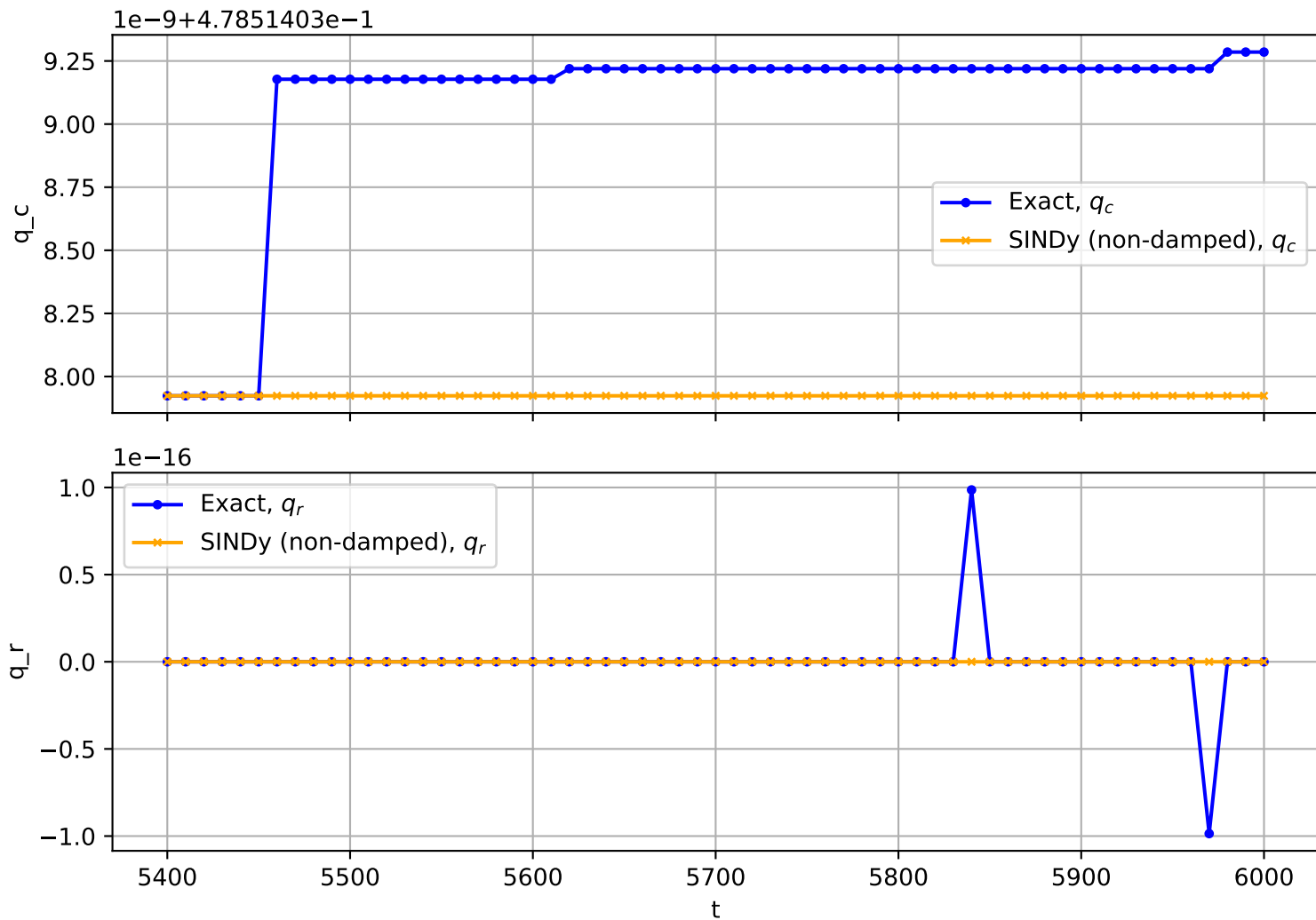
Trajectory No. 806
