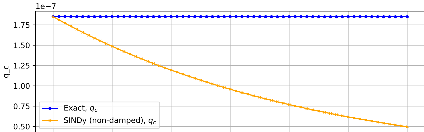
Trajectory No. 858
