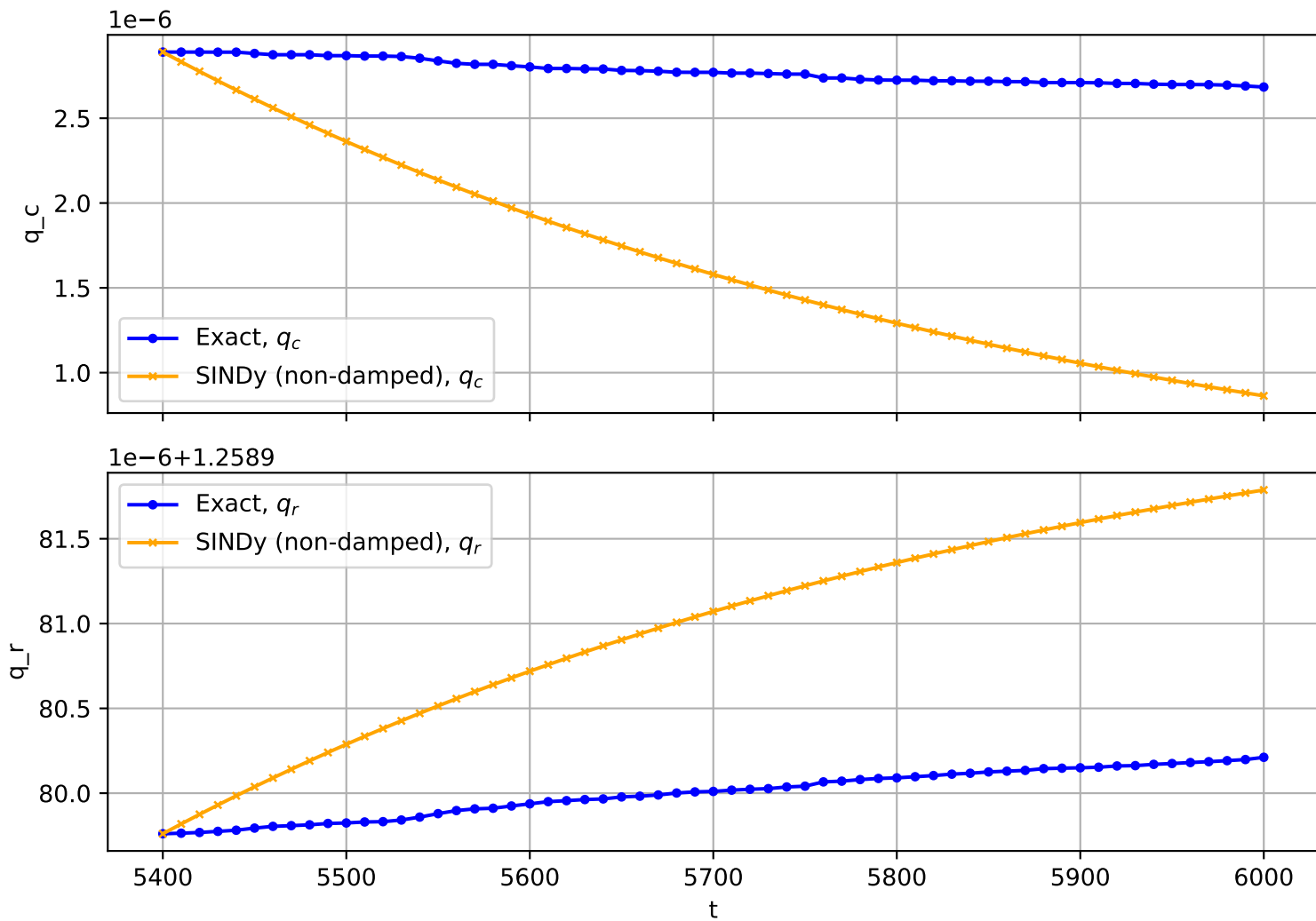
Trajectory No. 861
