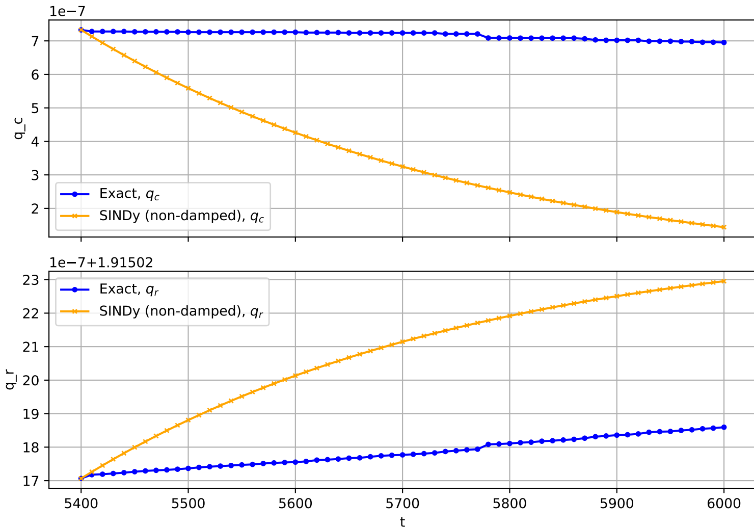
Trajectory No. 884
