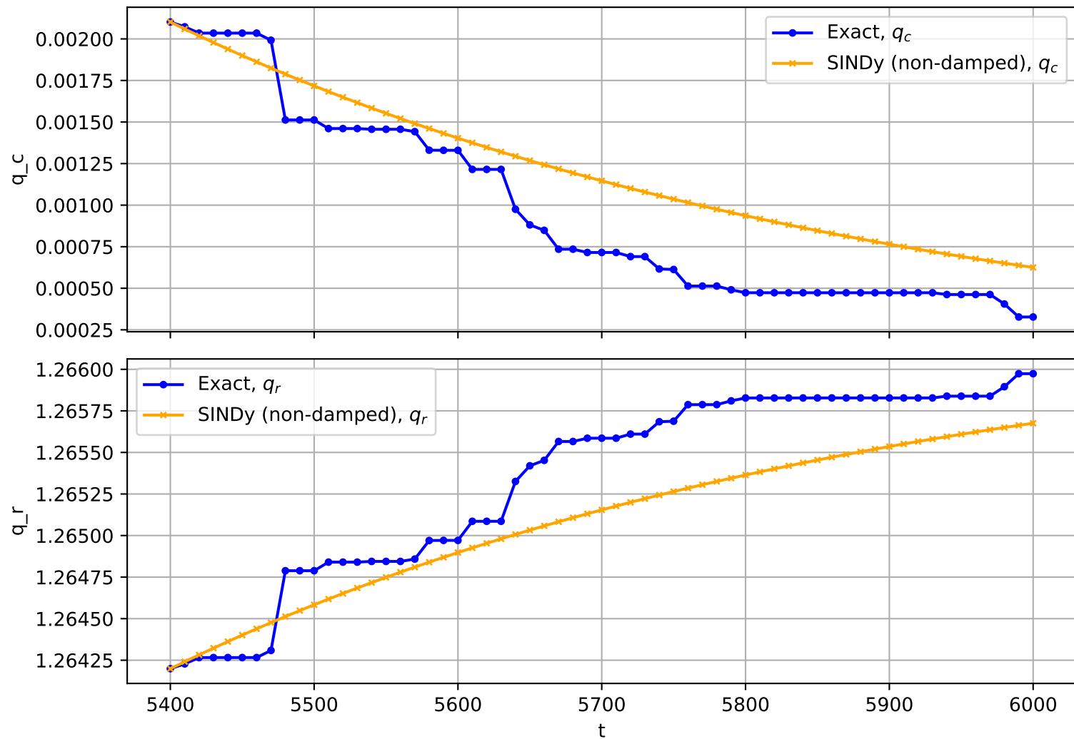
Trajectory No. 898
