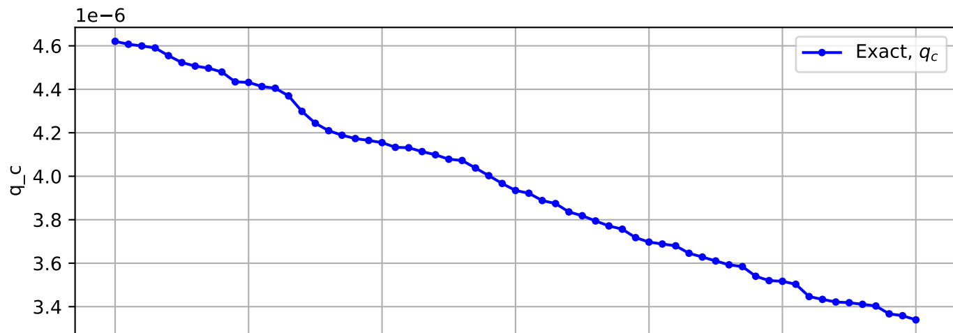
Trajectory No. 1068
