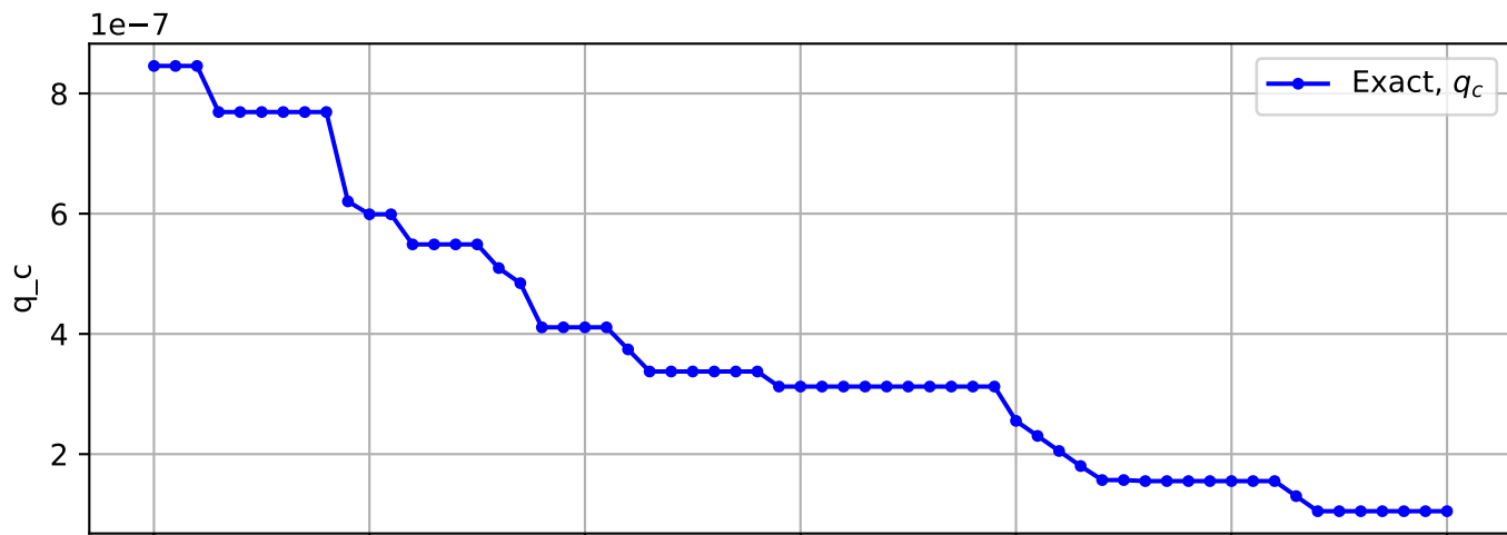
Trajectory No. 1087
