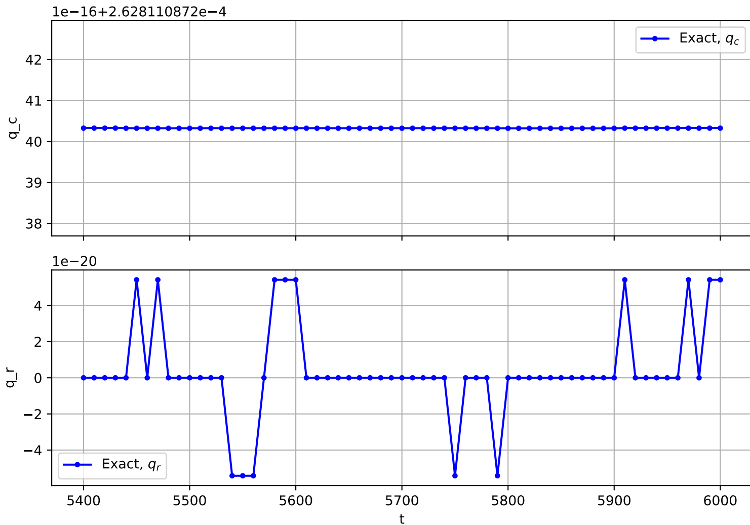
Trajectory No. 1136
