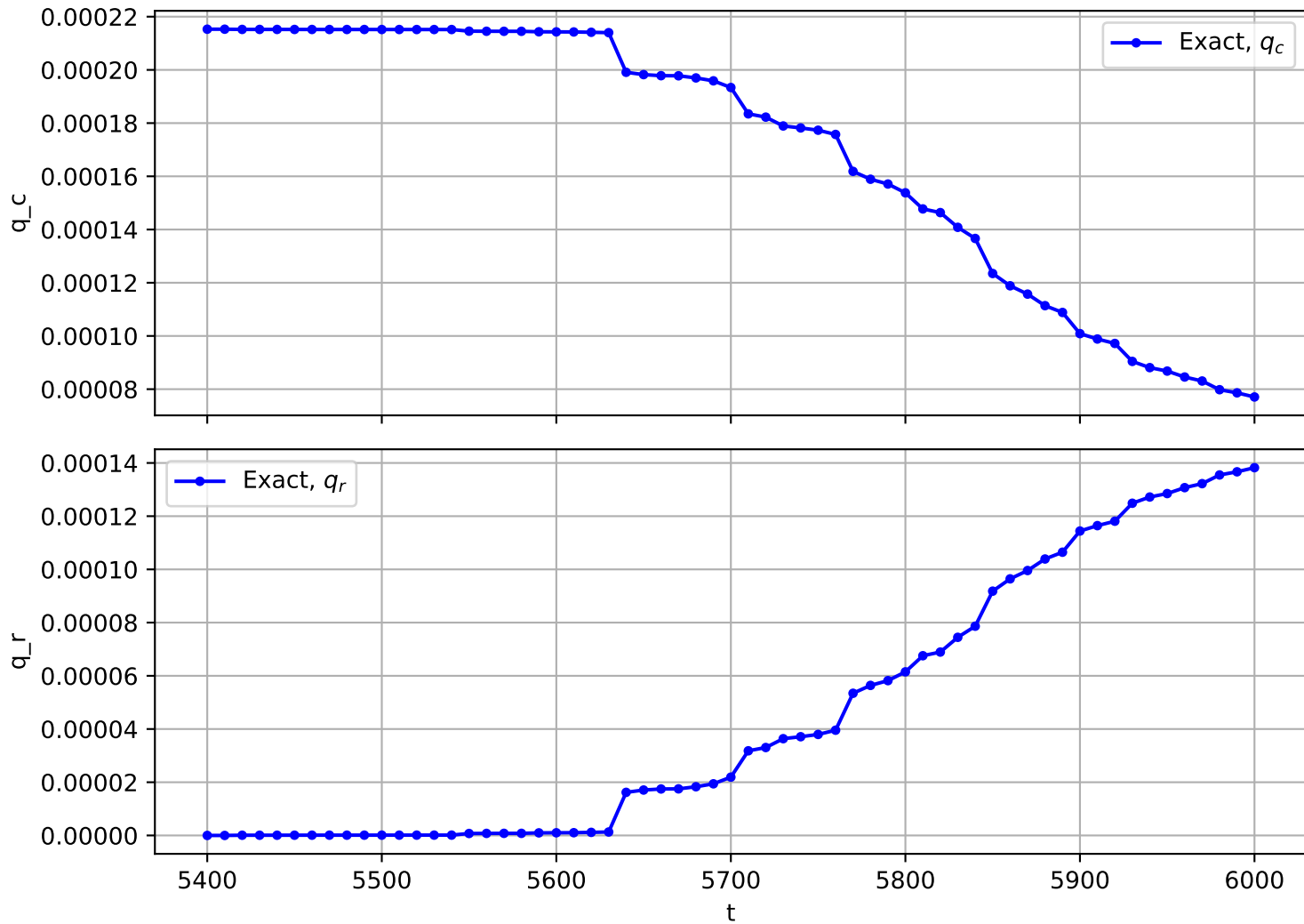
Trajectory No. 1142
