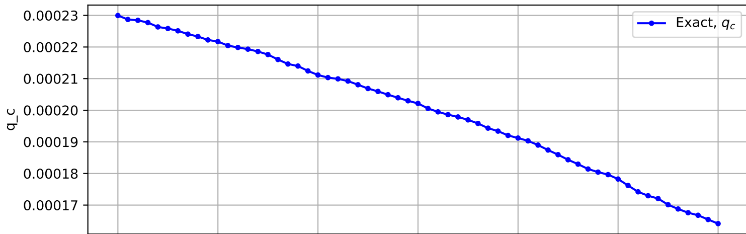
Trajectory No. 1158
