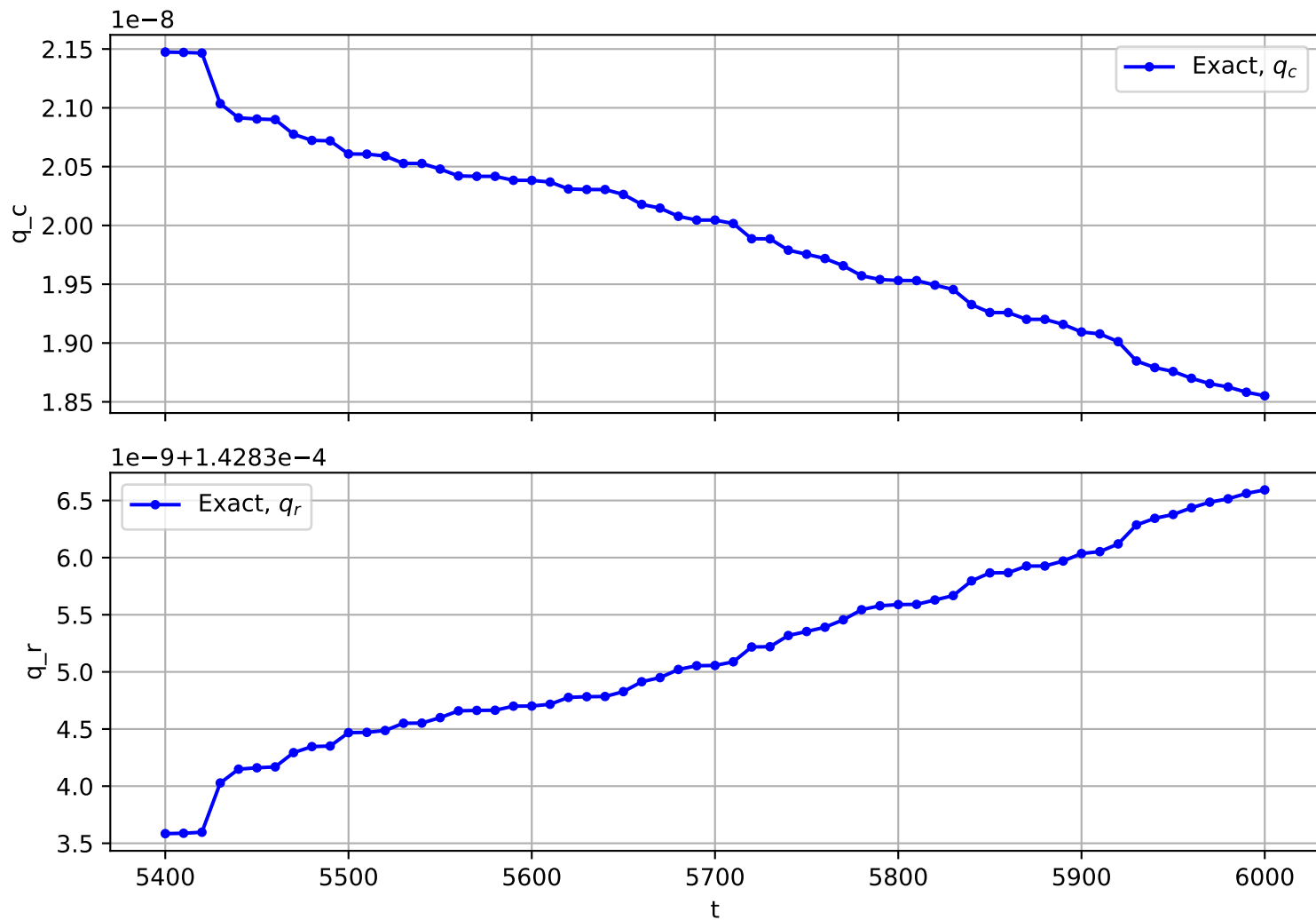
Trajectory No. 1188
