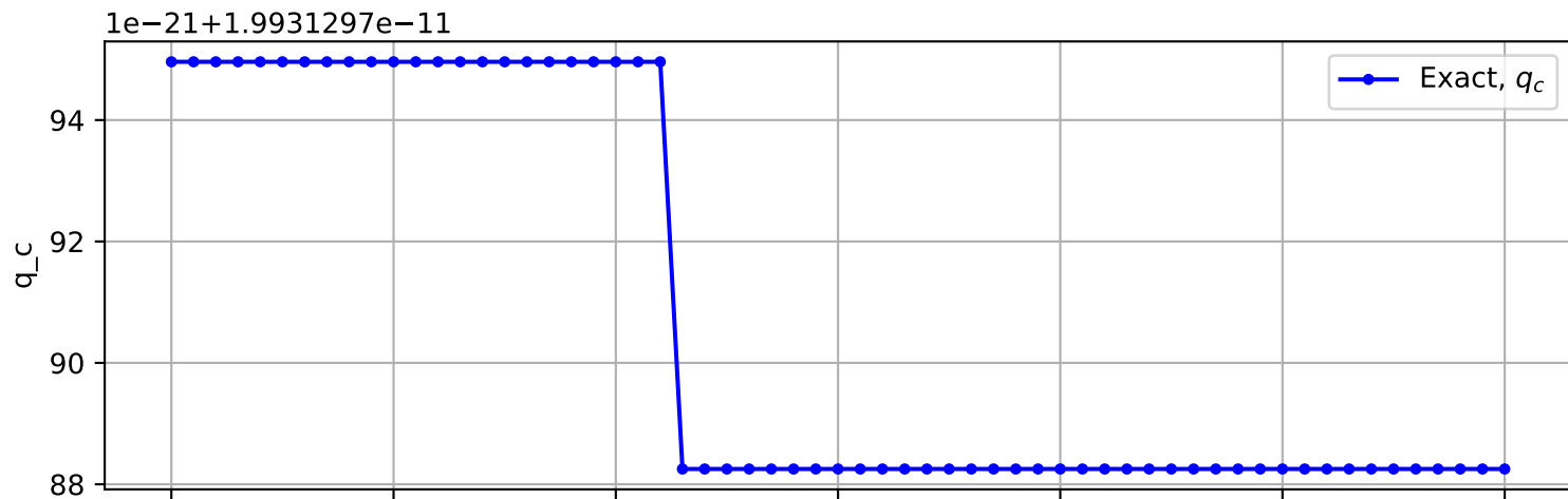
Trajectory No. 1300
