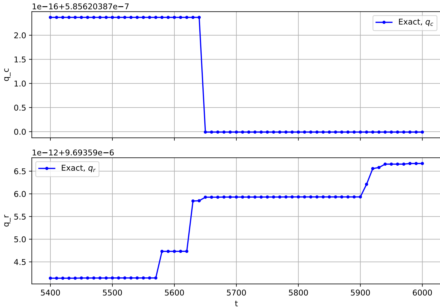
Trajectory No. 1381
