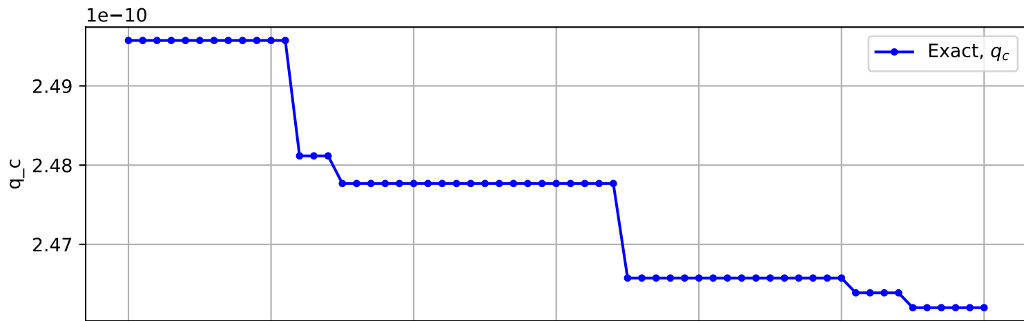
Trajectory No. 1415
