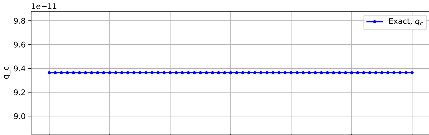
Trajectory No. 1435
