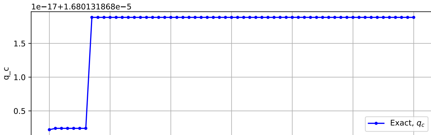
Trajectory No. 158
