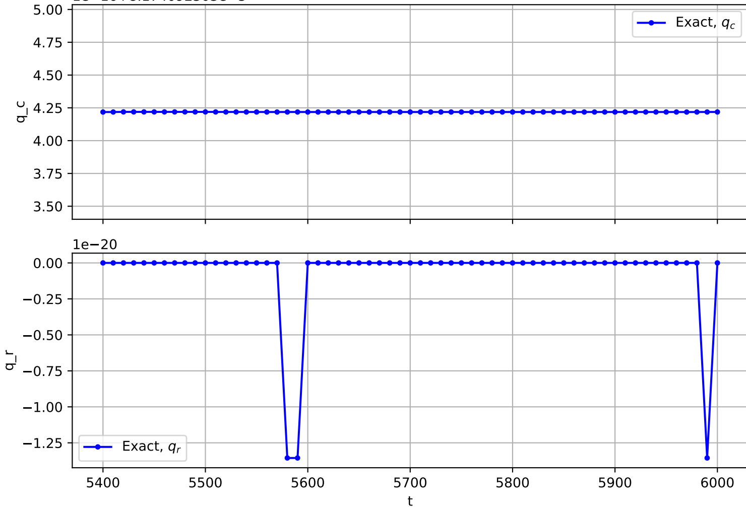
Trajectory No. 1619
