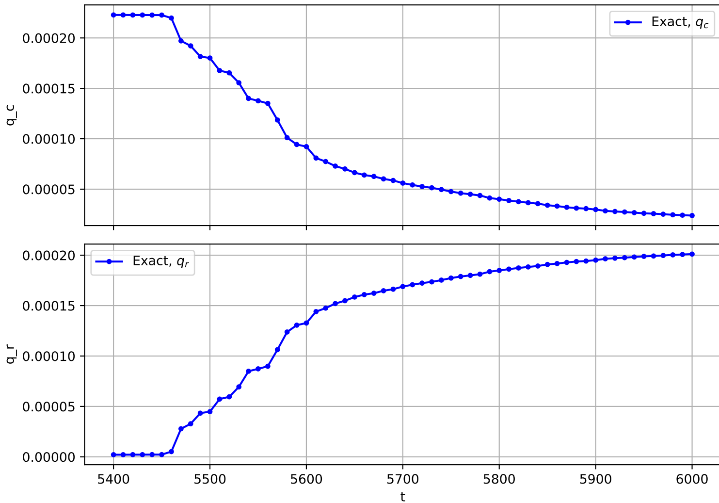
Trajectory No. 1735
