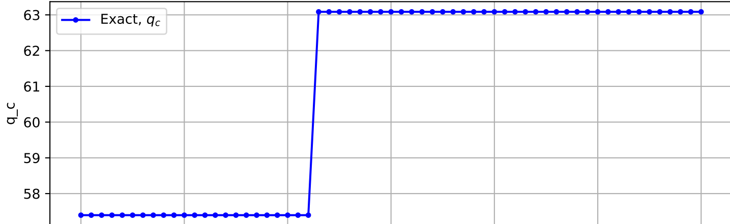
Trajectory No. 1787
