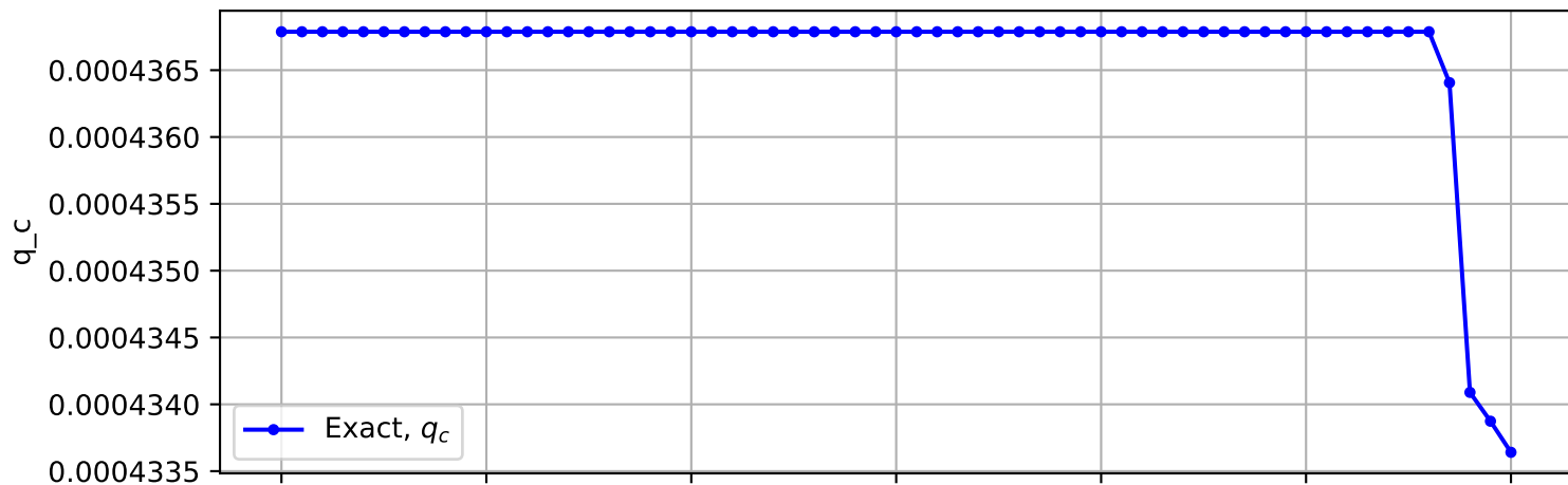
Trajectory No. 2036
