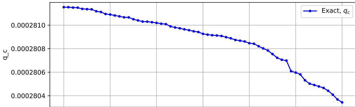
Trajectory No. 2052
