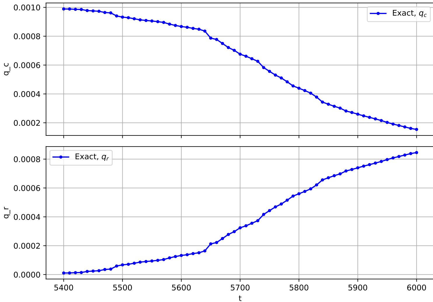
Trajectory No. 2111
