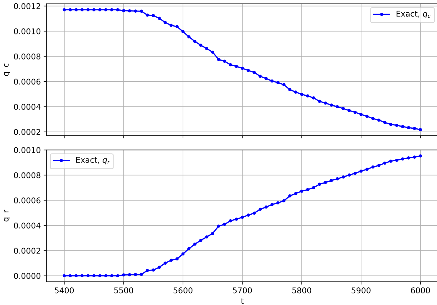
Trajectory No. 2149
