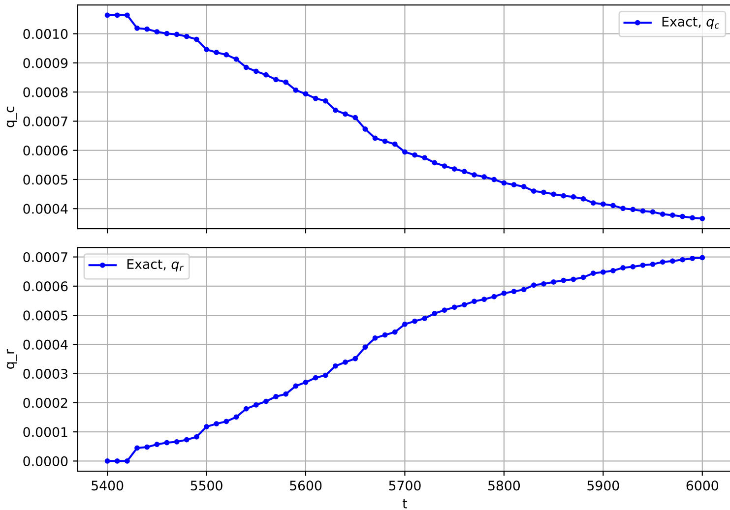
Trajectory No. 2158
