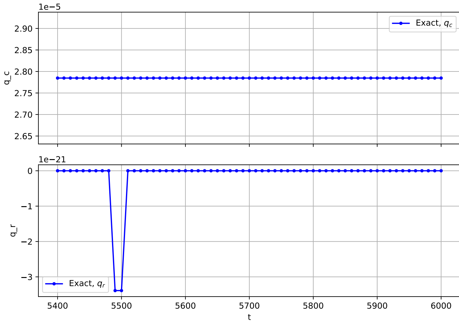
Trajectory No. 2170
