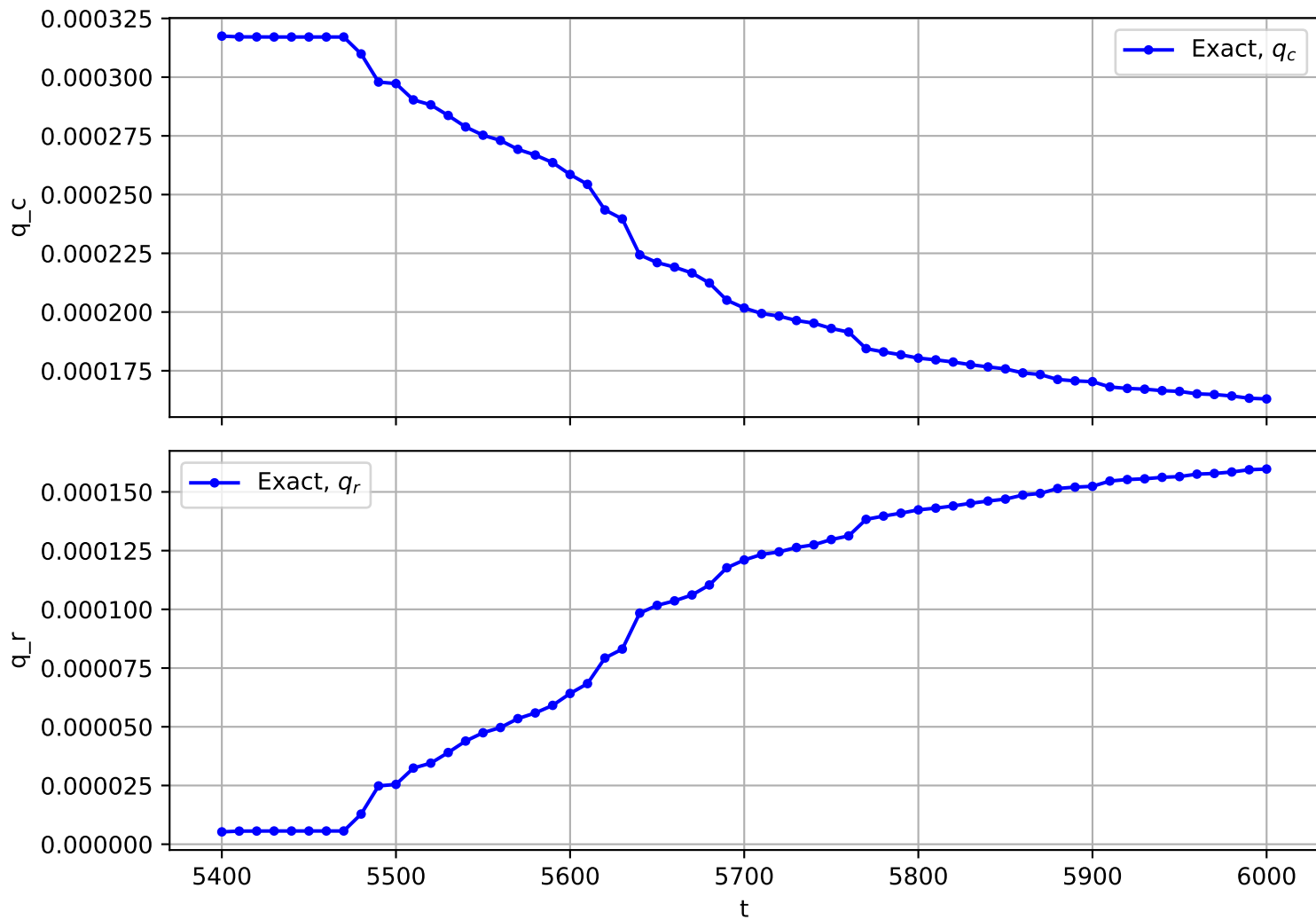
Trajectory No. 2174
