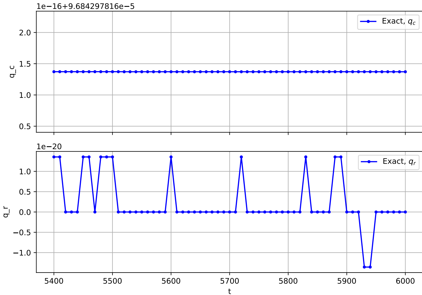
Trajectory No. 2176
