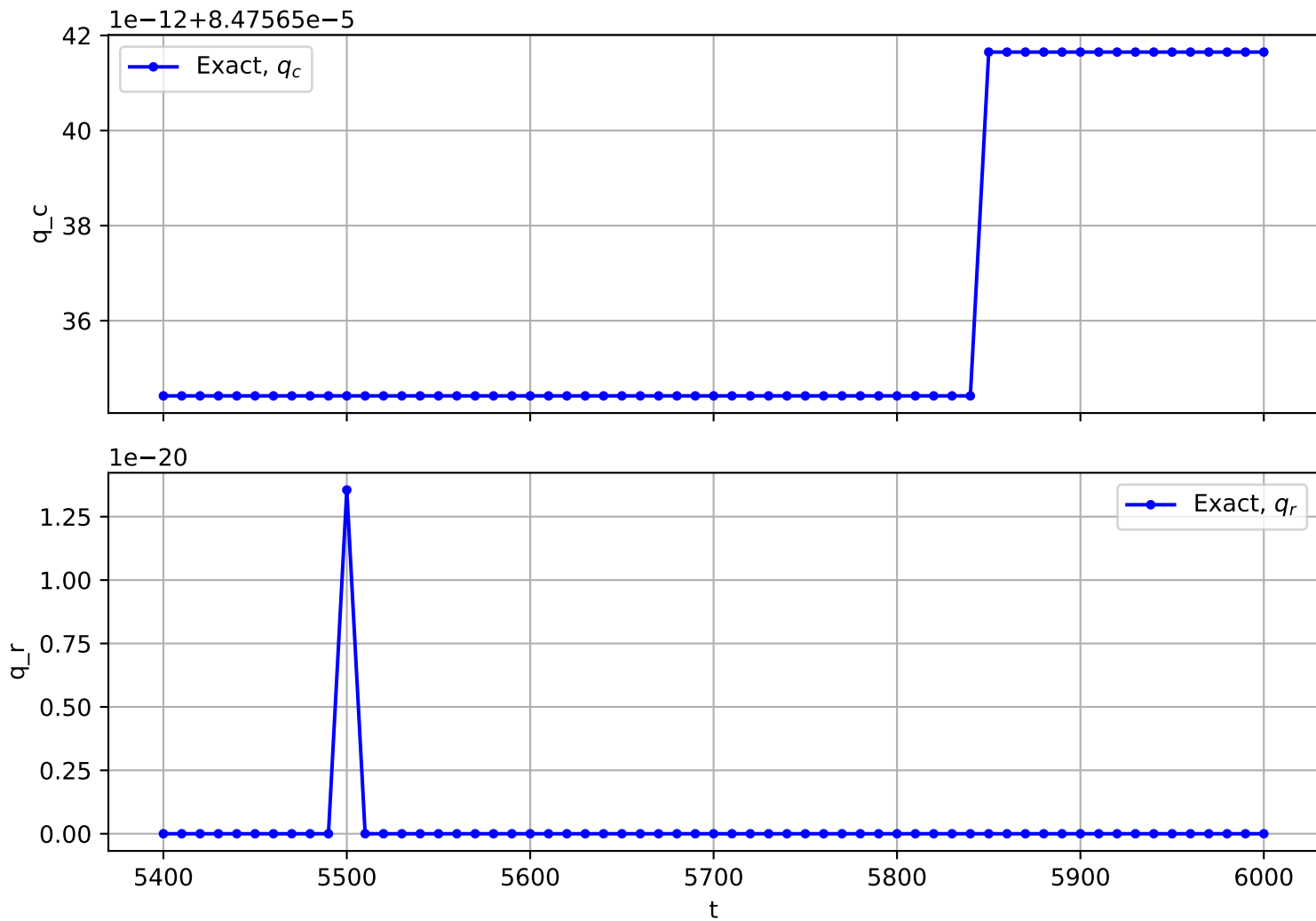
Trajectory No. 2240
