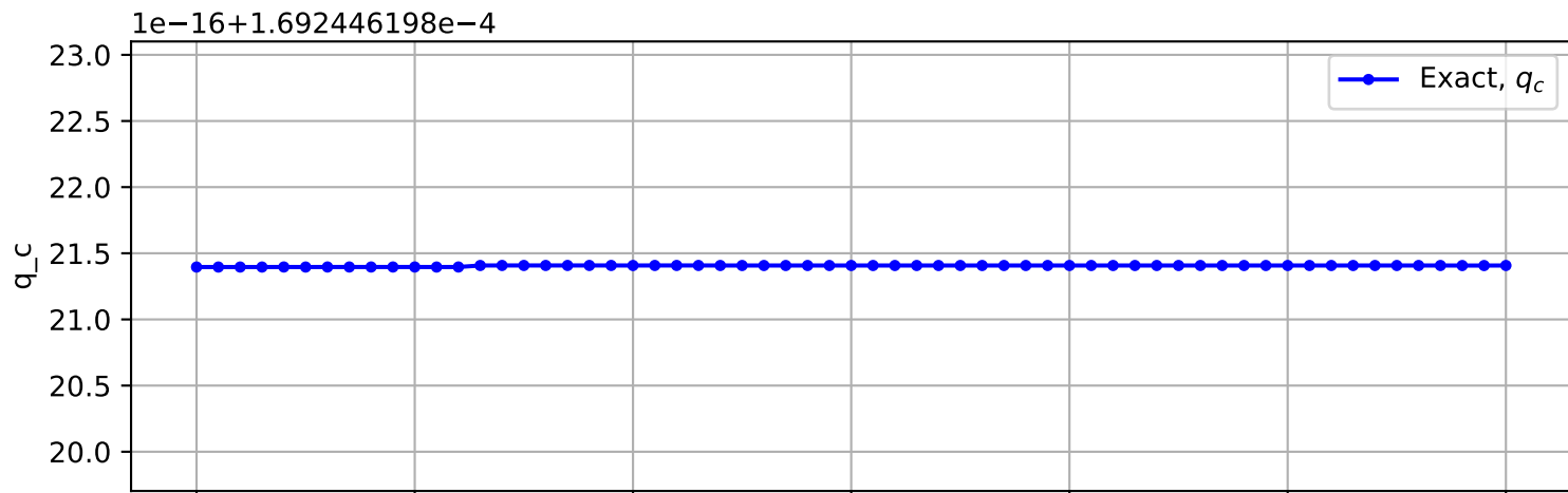
Trajectory No. 227
