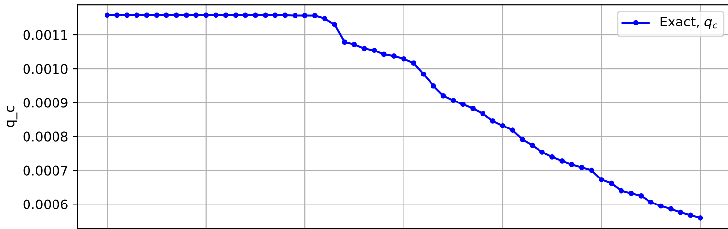
Trajectory No. 2299
