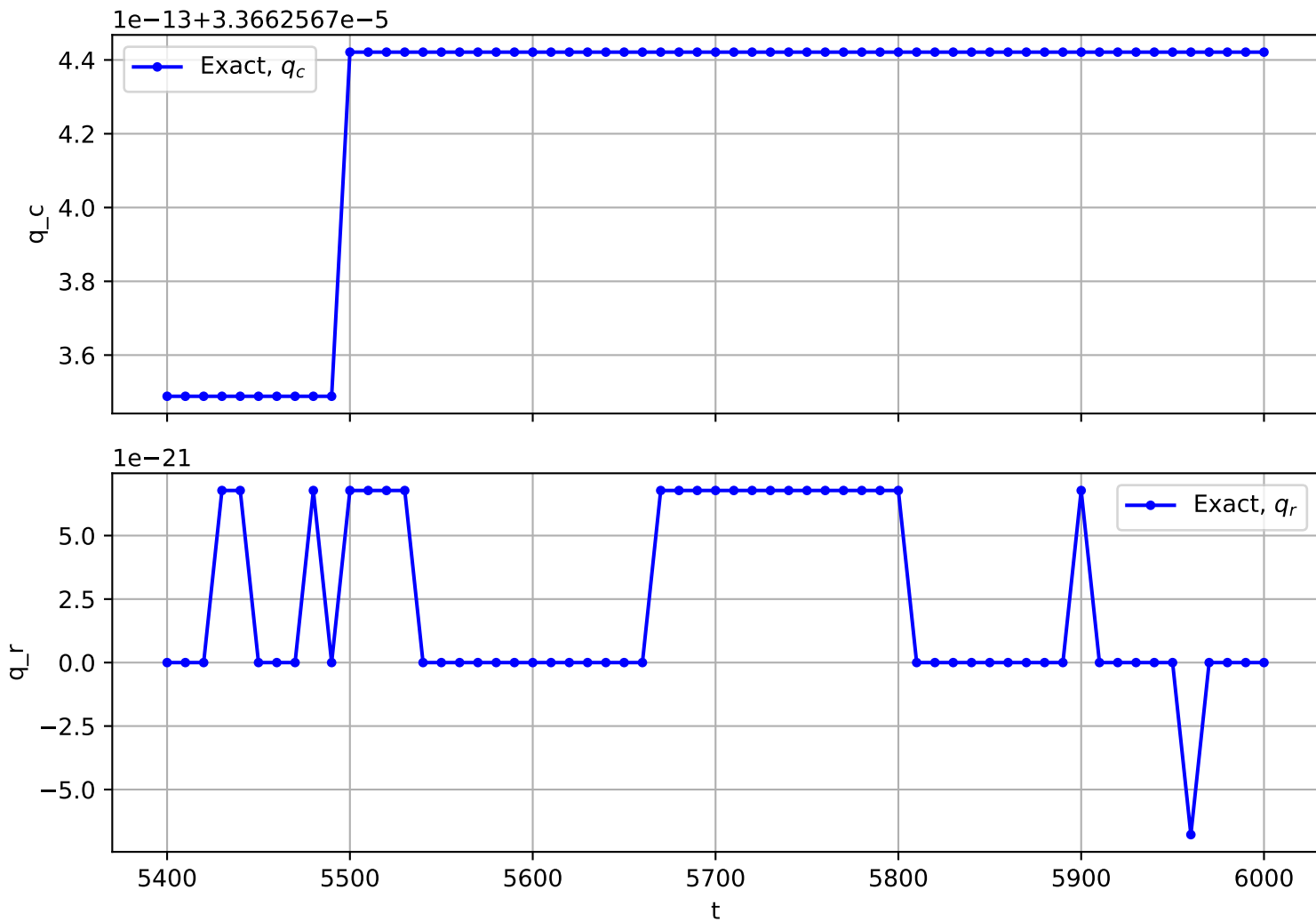
Trajectory No. 2313
