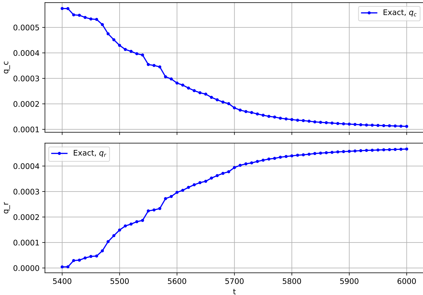
Trajectory No. 2316
