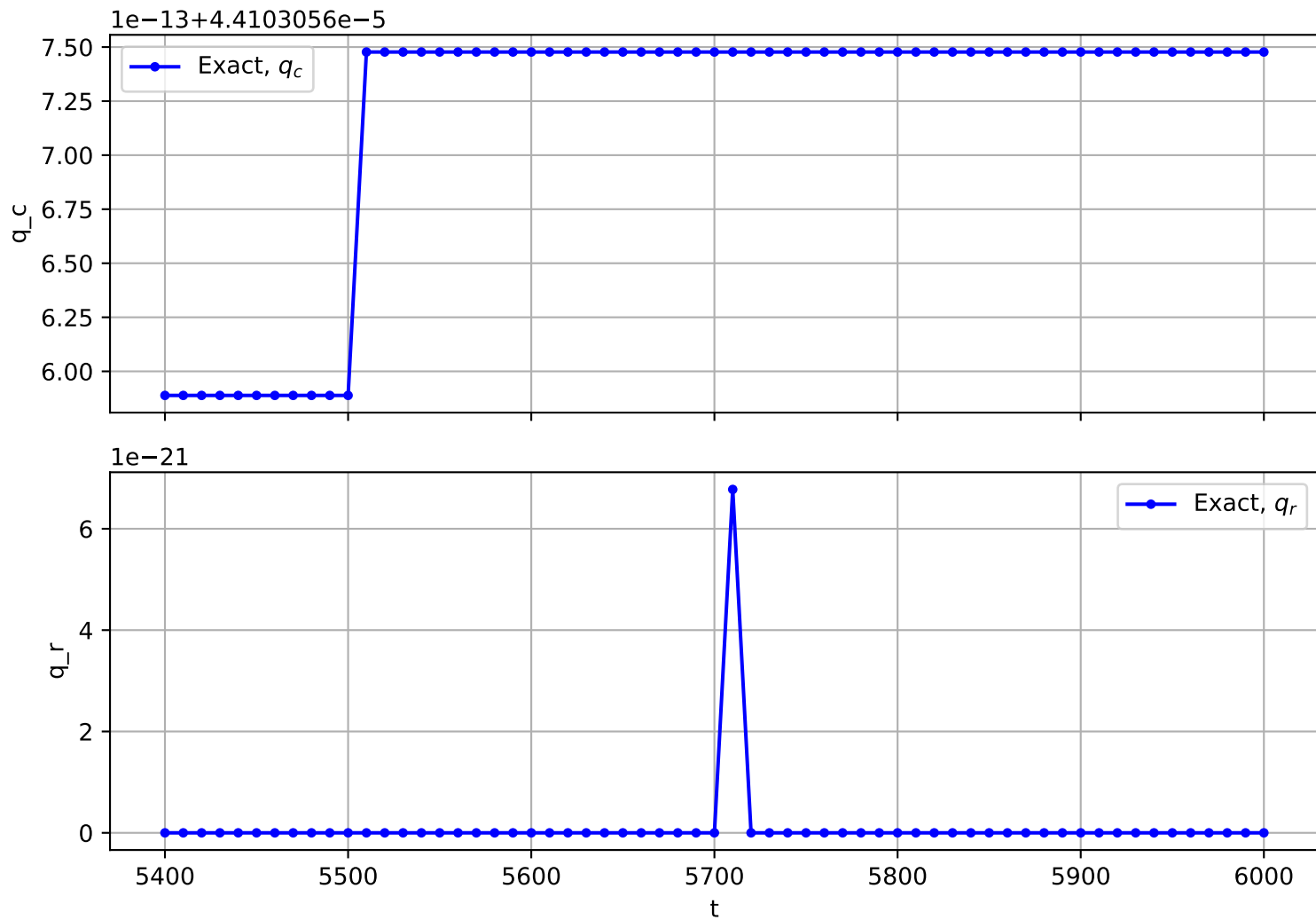
Trajectory No. 2320
