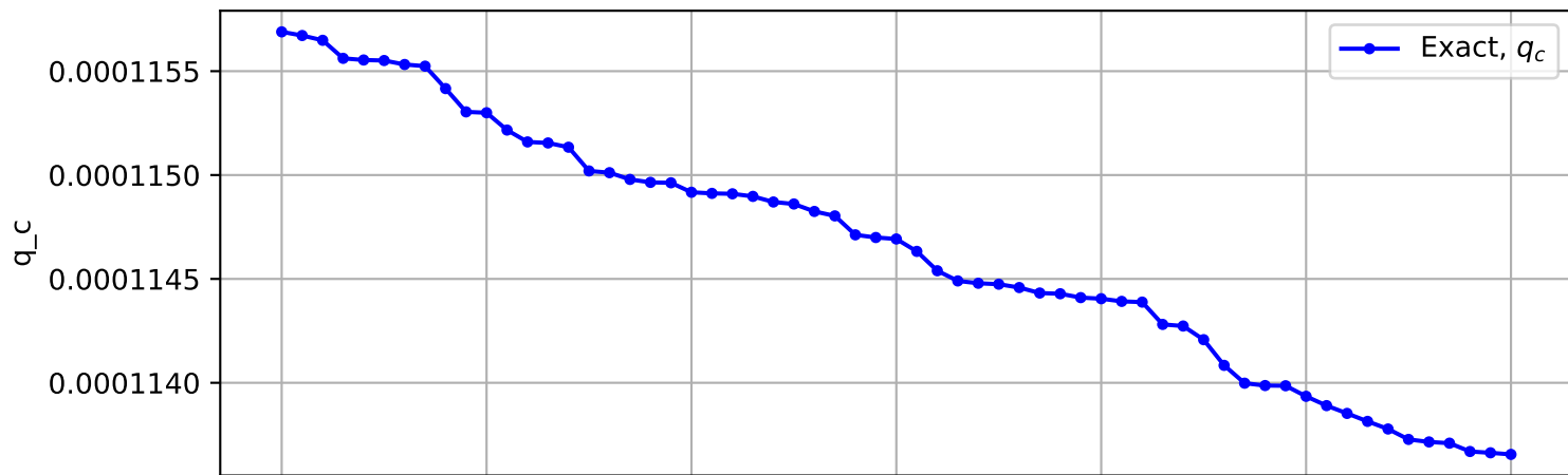
Trajectory No. 2327
