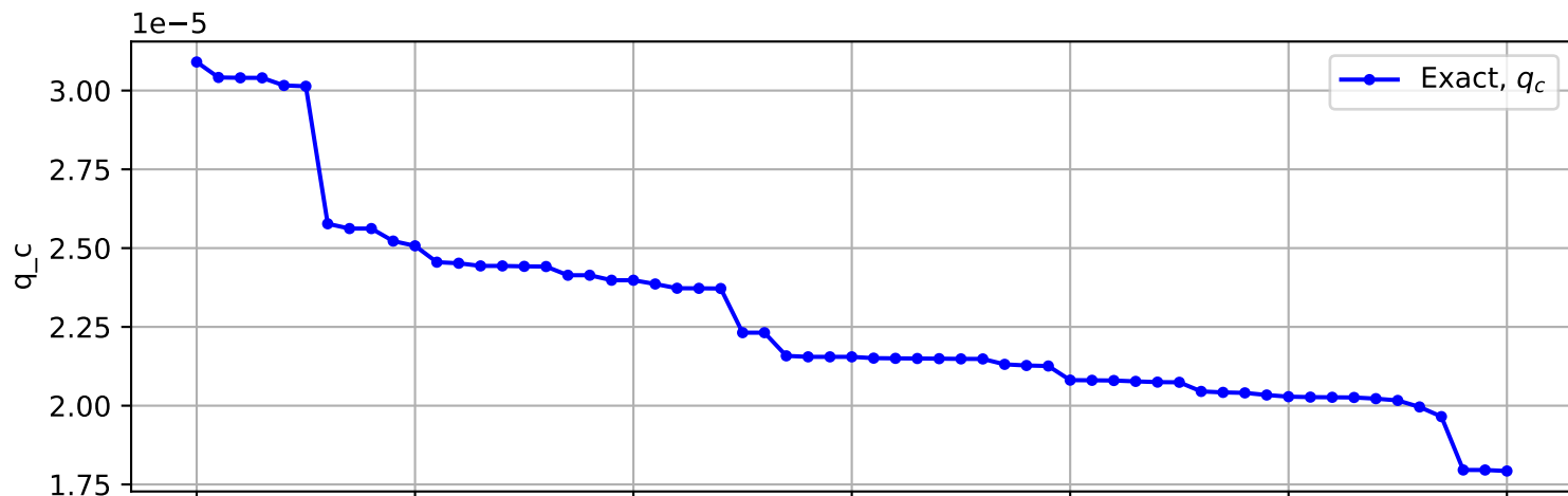
Trajectory No. 2351
